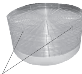
napájecí otvory
